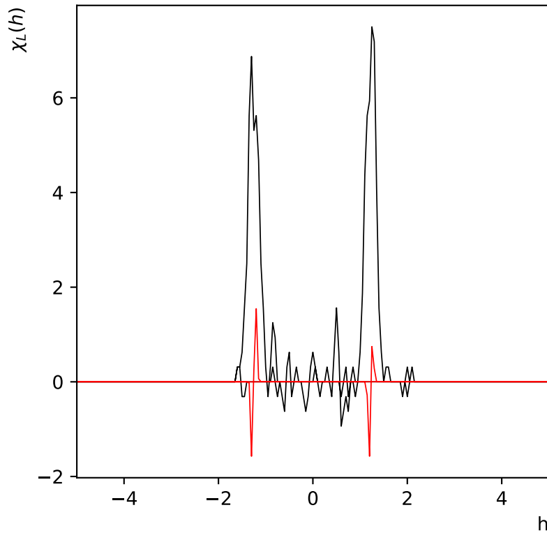
\chi_L(h) réseau de taille L=8 à T=1.5
