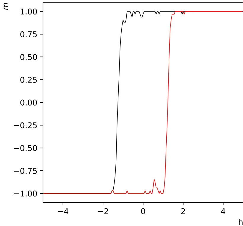
Hystérésis de l'aimantation réseau de taille L=8 - h=5 à T=1.5
